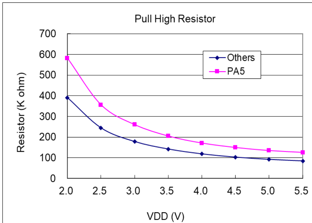
4.14. IO 引脚上拉/下拉阻抗曲线图
