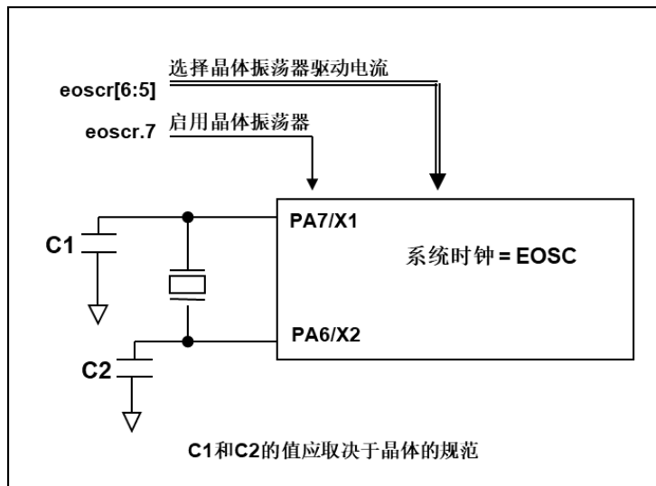
图 2: 晶体振荡器的硬件连接
