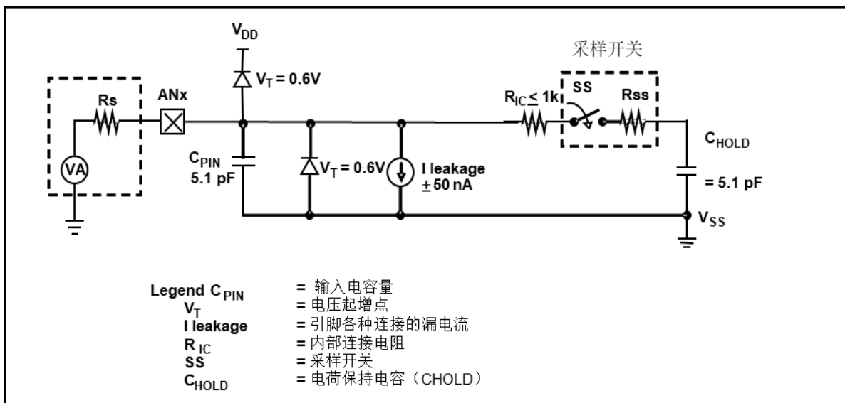
图 23：模拟输入模型
